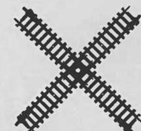
1856 90° Kreuzung, beide Stränge 115 mm.
